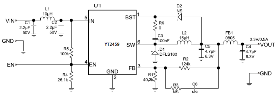
3.3V输出应用图
